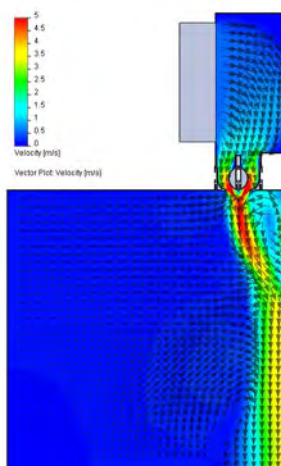
Jets d'air verticaux près de baies vitrées/cloisons
