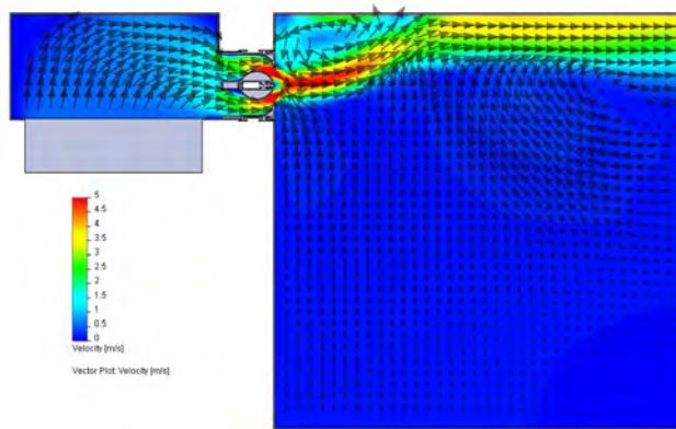
Jets d'air horizontaux avec montage mural
