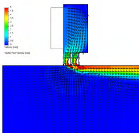
Jets d'air horizontaux à une direction
