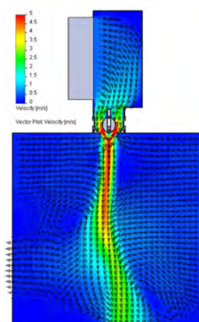
Jets d'air verticaux au centre de la pièce
