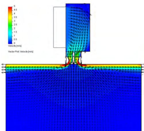
Jets d'air horizontaux dans deux directions opposées
